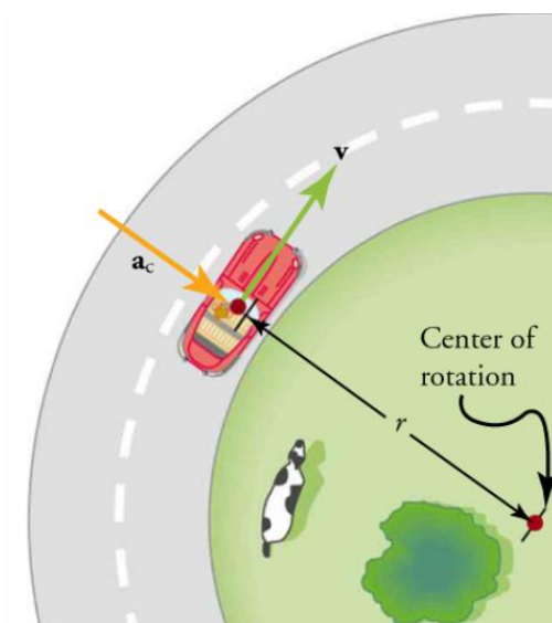
Figur 3.8: Bil svinger med sentripetalakselerasjon
