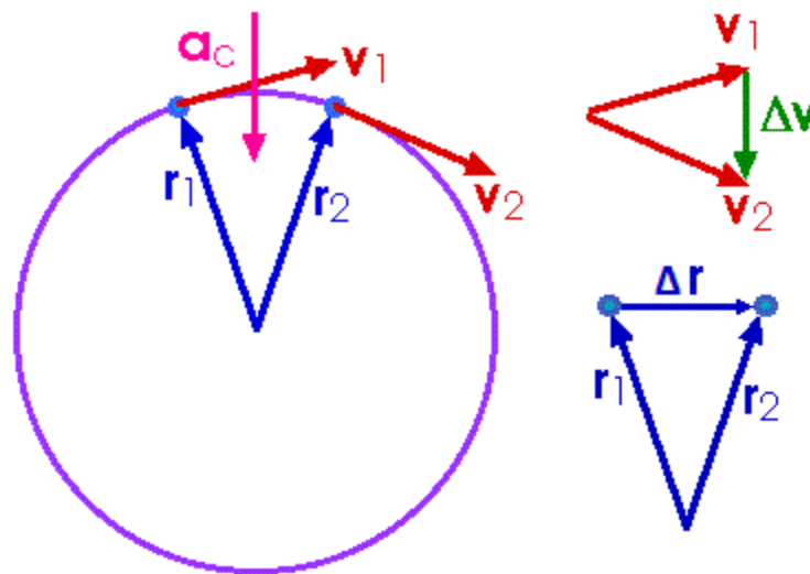
Figur 3.9: Utledning av sentripetalakselerasjon
