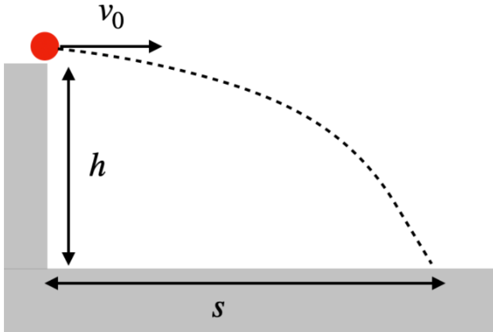
Figur 3.7: Ballen rett før den faller ut av klippen
