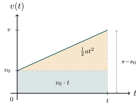
(b) v(t) -graf. Trapesarealet (rektangel + trekant) er forflytningen: \Delta s = s - s_0 .
